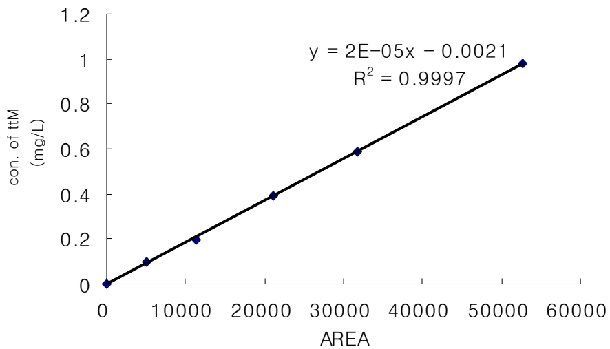
그림 2. trans,trans-muconic acid의 검량선
