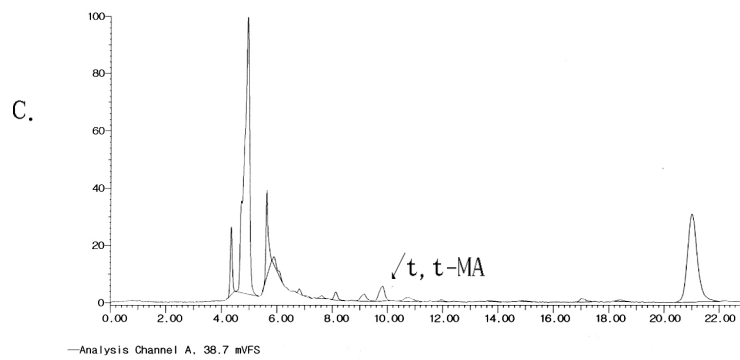
그림 1. t, t-MA의 크로마토그램. A, 표준물질의 크로마토그램; B, 소변시료의 크로마토그램; C, 표준물질을 첨가한 소변시료
